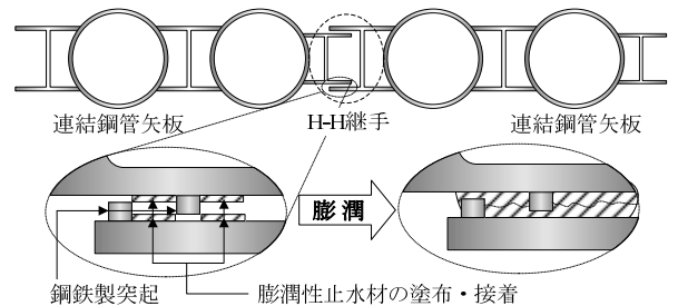
図-1 膨潤性止水材を用いたH-H継手の遮水処理
