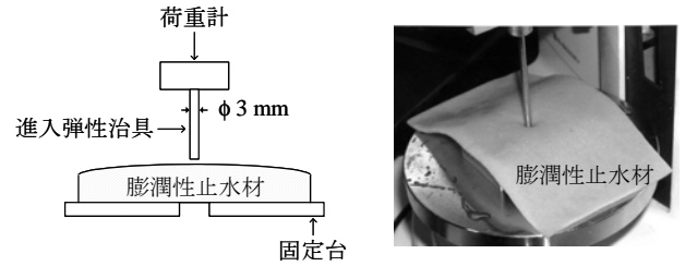
図-3 膨潤体膜強度試験の概要
