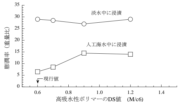
図-2 高吸収ポリマーのDS値と膨潤率
