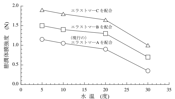
(b) 人工海水中に浸漬
