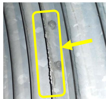
図6 現場施工後の膨潤状態
